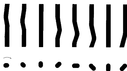
Rys. 41 Schemat ilustrujący charakter obserwowanych niestabilności strugi zimnej cieczy w przekroju pionowym kanału walcowego.
