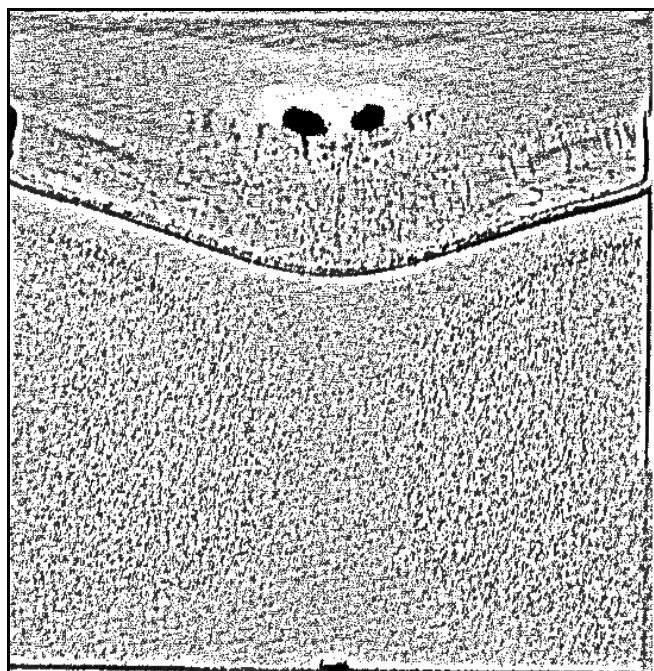
Rys. 9. Operacja przygotowująca obrazy do procesu korelacji PIV. Obraz zawiesziny ciekłokrystalicznej (Rys. 7) po filtracji pozwalającej na jednorodne uwypuklenie struktury posiewu.
