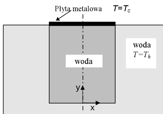
Rys. 1. Schemat ideowy badanych kanałów z izotermiczną ścianką górną o temperaturze T_c i pozostałych ściankach nie-adiabatycznych, opływanych cieczą o stałej temperaturze T_h .
