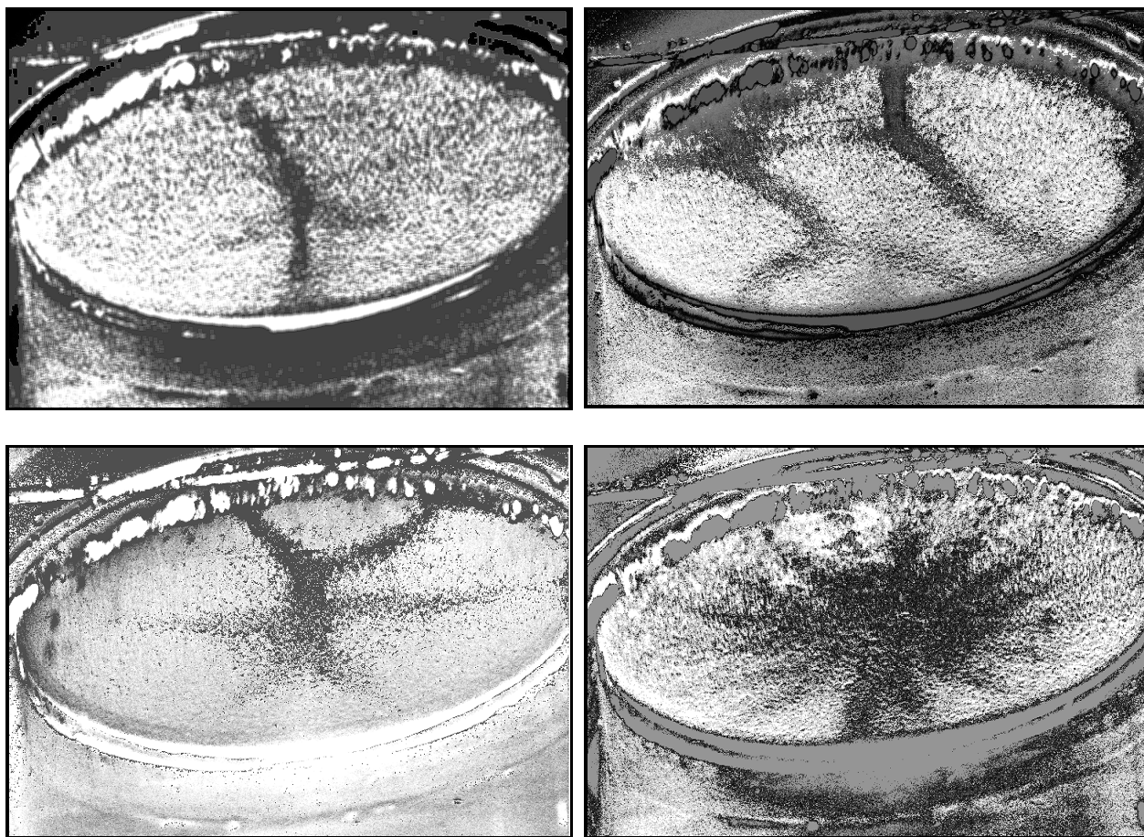
Rys. 42. Niestabilności struktury przepływu w kanale walcowym (W1); T_h=25^{\circ}\text{C} , T_c=-10^{\circ}\text{C} . Fluktuacje pola temperatury obserwowane pod górną powierzchnią widoczne w postaci zmian zabarwienia zawiesiny ciekłokrystalicznej. Ciemny kolor (czerwony) odpowiada niższej temperaturze.
