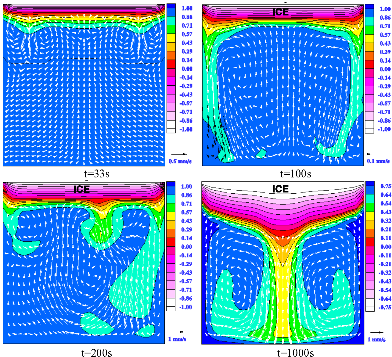
Rys. 19. Rozwój przepływu w kanale sześciennym o ściankach szklanych, T_h=10^\circ\text{C} , T_c=-10^\circ\text{C} . Rezultaty obliczeń dla 33s, 100s, 200s i 1000s od „ciepłego startu” pokazujące bezwymiarowe izotermie i pole prędkości dla centralnego przekroju pionowego.
