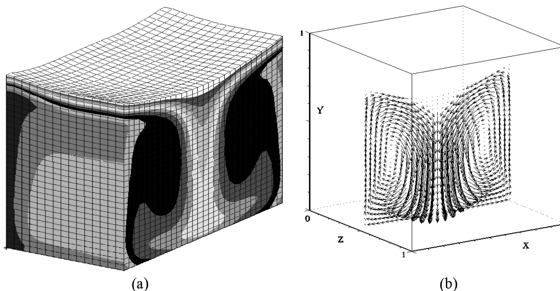
Rys. 17. Rezultaty obliczeń dla kanału z pleksiglasu, T_h=20^{\circ}\text{C} , czas t=1000\text{s} od „zimnego startu”; (a) - siatka obliczeniowa i izotermy dla ciekowej domeny obliczeniowej (pokazany przekrój centralny dla połowy kanału) , (b) - pole wektorowe prędkości dla centralnego przekroju pionowego.
