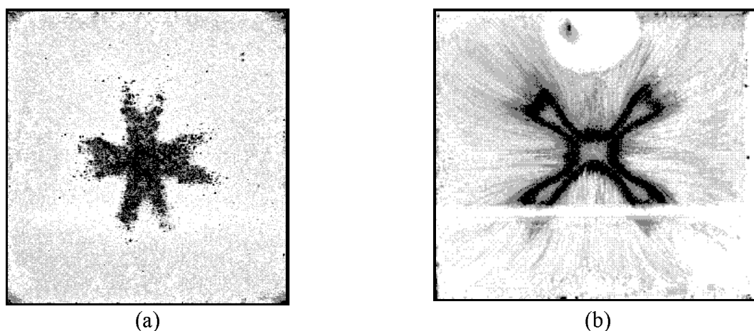
Rys. 34. Rozkład temperatury rejestrowany przy pomocy zawiesiny ciekłokrystalicznej w pobliżu górnej ścianki kanału sześciennego; (a) - 8mm ścianka boczna z pleksiglasu (P) ; (b) - 2mm ścianka ze szkła (S). Ciemniejsze zabarwienie (kolor czerwony) odpowiada niższej temperaturze (por. Rys. A 2).
