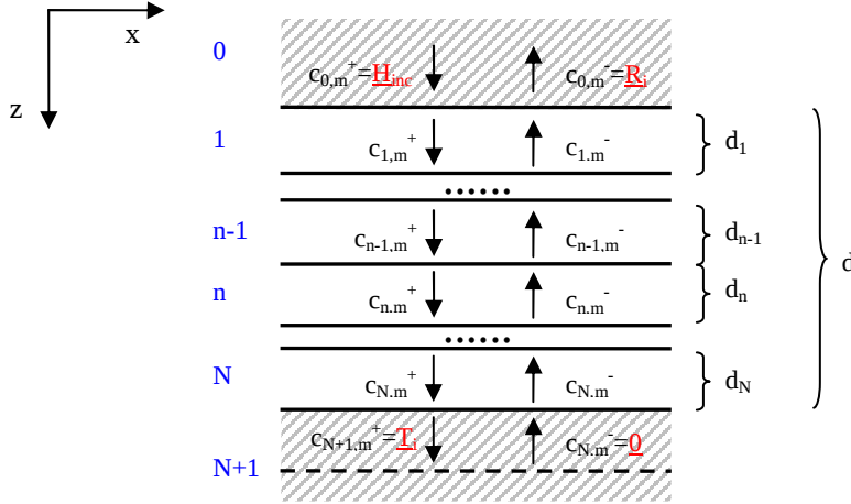
Rysunek 5.2. Schematyczne przedstawienie siatki dyfrakcyjnej o N warstwach z zaznaczonymi modami wewnątrz struktury oraz rzędami ugięcia na zewnątrz. Obszary zakreskowane są zewnętrznymi dielektrycznymi obszarami jednorodnymi. Przerwana linia oznacza granicę numeryczną, która może być położona arbitralnie blisko granicy między obszarami N i N+1 , na podst. [76].
