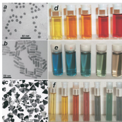
Rysunek 1.2. Lewa kolumna: Wizualizacja nanocząstek metali za pomocą elektronowej mikroskopii transmisyjnej: (a) złote nanosfery, (b) złote nanopręciki, (c) srebrne nanoprismy. Prawa kolumna: Roztwory koloidalne: (d) nanocząstek stopów złota i srebra o rosnącej koncentracji złota, (e) złote nanopręciki o rosnącym stosunku długości do szerokości, (f) srebrne nanoprismy o rosnących wymiarach poprzecznych [37].
