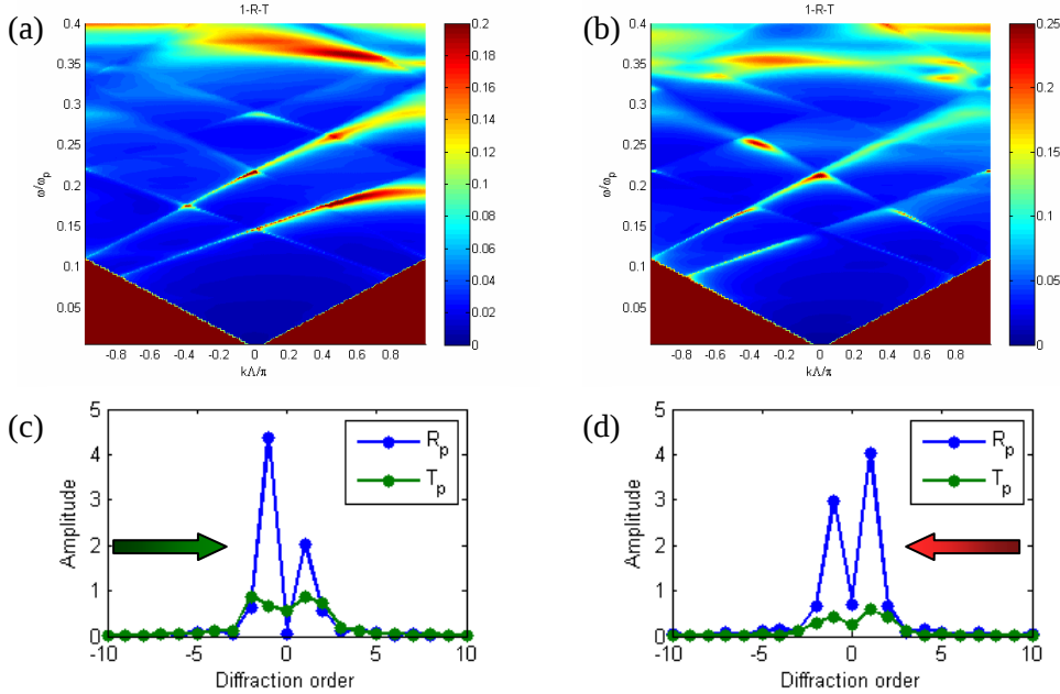
Rysunek 6.4. (a) i (b) Relacje dyspersji asymetrycznej dwuwarstwowej struktury o parametrach: \Lambda = 619nm , d_1 = 51nm , d_2 = 75nm , f_1 = 0.381\Lambda , f_2 = 0.421\Lambda , n_4 = 1 , n_5 = 1.5 oraz (c) i (d) unormowane amplitudy kolejnych rzędów ugięcia pola H_y dla d_x = 0.148\Lambda (lewa kolumna) i d_x = 0.35\Lambda (prawa kolumna).
