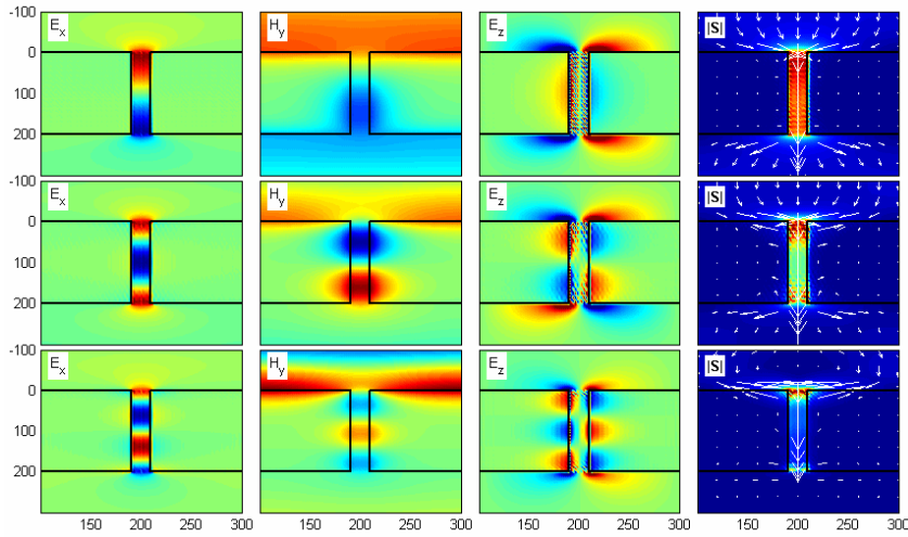
Rysunek 7.19. Rozkłady unormowanych amplitud składowych pól E_x , H_y i E_z oraz wartość ikierunek wektora Poyntinga dla trzech najniższych rzędów rezonansów wnękowych dla częstotliwości: \omega = 0.169\omega_p , \omega = 0.315\omega_p , \omega = 0.419\omega_p . Okres siatki \Lambda = 200nm , grubość d = 200nm , wypełnienie struktury f = 0.9\Lambda , jednorodne, symetryczne otoczenie dielektryczne ( n_1 = n_4 = n_3 = 1 ).
