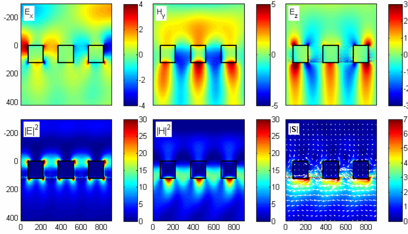
Rysunek 7.23. Niezerowe składowe pól, ich natężenia oraz amplituda i kierunek wektora Poyntinga dla dyspersyjnego modu na siatce o okresie \Lambda = 300\text{nm} , wypełnieniu f = 0.5\Lambda , wysokości d = 120\text{nm} . Częstotliwość fali: \omega = 0.255\omega_p , k = 0.28\pi/\Lambda ( \theta = 14.5^\circ ), współczynniki załamania: n_1 = n_4 = 1 , n_3 = 1.5 .
