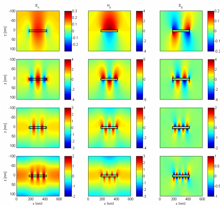
Rysunek 7.10. Unormowane amplitudy składowych E_x , H_y i E_z dla czterech pierwszych nieparzystych rezonansów dla grubości siatki d=10nm w jednorodnym, symetrycznym otoczeniu dielektrycznym ( n_1 = n_4 = n_3 = 1 ). Okres: \Lambda = 600nm , wypełnienie struktury f = 0.4\Lambda .
