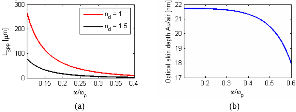
Rysunek 4.4. (a) Długość drogi propagacji plazmonu polarytonu powierzchniowego na styku złota i dielektryka w zależności od częstotliwości fali padającej dla \epsilon_d = 1 oraz \epsilon_d = 2.25 . b) Głębokość wnikania pola elektromagnetycznego SPP w złoto w zależności od częstotliwości fali padającej.
