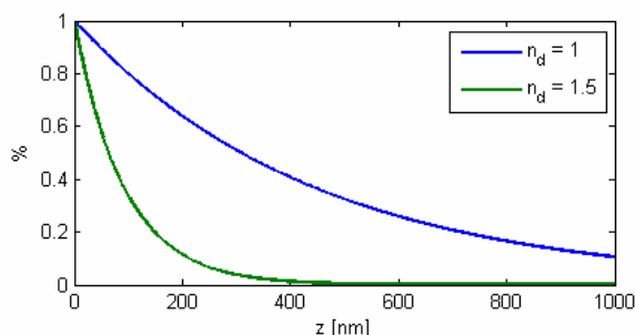
Rysunek 7.5. Amplituda pola plazmonu w dielektryku, w kierunku prostopadłym do granicy z metalem w zależności od odległości od granicy w różnych dielektrykach o współczynnikach załamania n_d = 1 i n_d = 1.5 .
