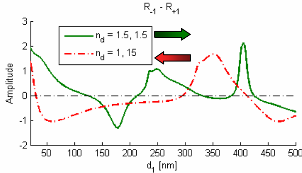
Rysunek 6.13. Różnica modułów amplitud -1 i +1 odbitego rzędu ugięcia w zależności od grubości górnej siatki d_1 . Zielona ciągła linia: struktura o współczynnikach n_3 = n_4 = n_5 = 1.5 , dla zoptymalizowanych parametrów kierująca energię w prawo, czerwona przerywana linia: struktura o współczynnikach n_3 = n_5 = 1.5 , n_4 = 1 , dla zoptymalizowanych parametrów kierująca energię w lewo. Pozostałe parametry są stałe dla obu konfiguracji: \lambda = 632.8\text{nm} , \Lambda = 624\text{nm} , d_x = 0.35\Lambda , f_1 = 0.372\Lambda , f_2 = 0.443\Lambda , d_2 = 70\text{nm} .
