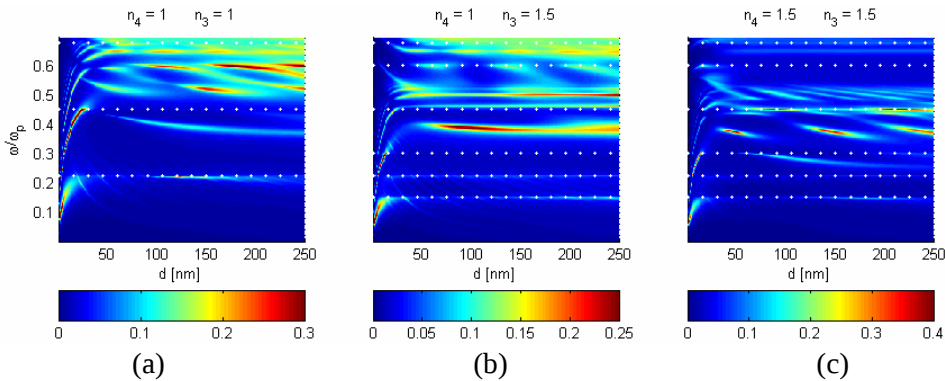
Rysunek 7.24. Absorpcja dla pojedynczej siatki w zależności od jej grubości, (a) n_4 = 1 , n_3 = 1 , (b) n_4 = 1 , n_3 = 1.5 , (c) n_4 = 1.5 , n_3 = 1.5 . Pozostałe parametry: \Lambda = 600\text{nm} , f = 0.4\Lambda .
