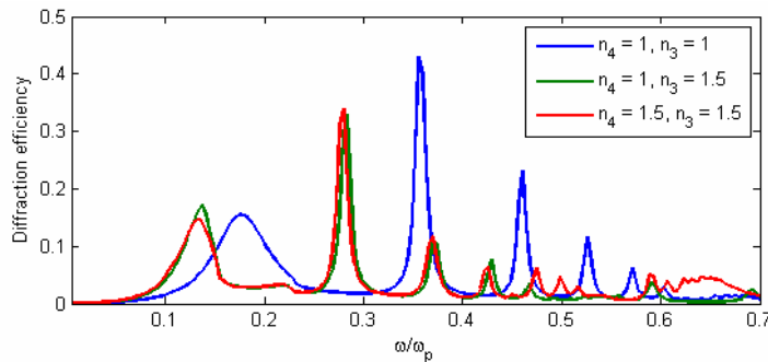
Rysunek 7.25. Zmiana położenia pików rezonansowych w zależności od częstości fali padającej dla siatek o grubości d = 10nm i różnych współczynnikach załamania otoczenia. Pozostałe parametry: \Lambda = 600nm , f = 0.4\Lambda .
