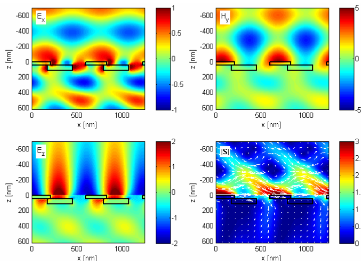
Rysunek 6.9. Unormowane amplitudy niezerowych składowych pola elektromagnetycznego: E_x , H_y , E_z oraz wartość i kierunek wypadkowego wektora Poyntinga |\underline{S}| w pobliżu asymetrycznej dwuwarstwowej struktury o parametrach: d_x = 0.35\Lambda , \Lambda = 624\text{nm} , d_1 = 46\text{nm} , d_2 = 70\text{nm} , f_1 = 0.372\Lambda , f_2 = 0.443\Lambda , n_4 = n_5 = 1.5 .
