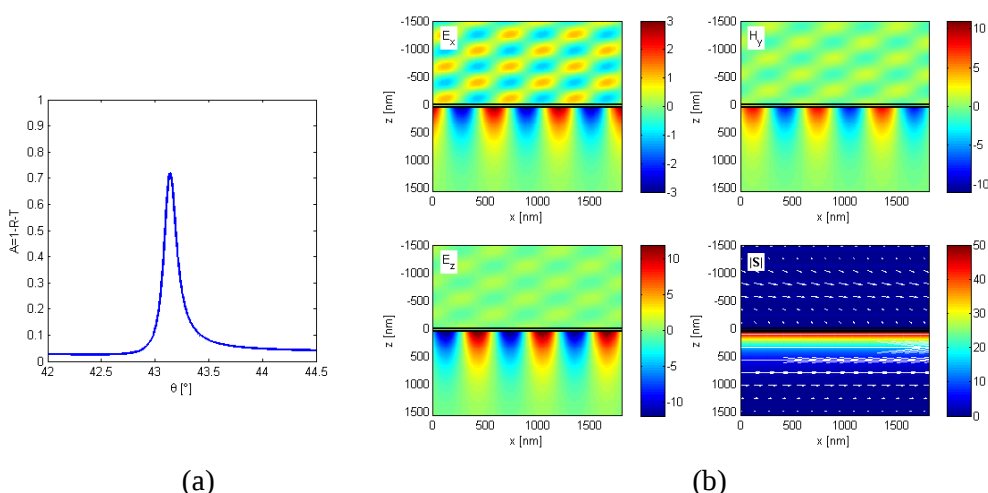
Rysunek 7.4. (a) Absorpcja warstwy metalu o grubości d = 60\text{nm} w zależności od kąta padania fali płaskiej o długości \lambda = 632.8\text{nm} w konfiguracji Kretschmanna ( \epsilon_1 = 2.25 , \epsilon_3 = 1 ). (b) Rozkład niezerowych składowych pola EM oraz wektora Poyntinga dla rezonansowego kąta padania ( \theta = 43.14^\circ ).
