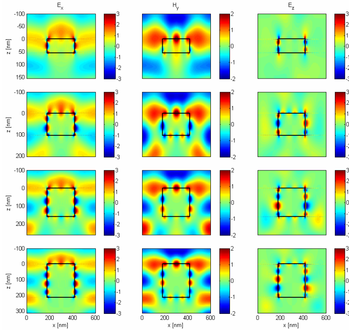
Rysunek 7.16. Rozkłady unormowanych amplitud składowych pól E_x , H_y i E_z dla kolejnych rezonansów przy rosnącej grubości siatki ( d = 53.7\text{nm} , 104\text{nm} , 160\text{nm} , 211\text{nm} ) dla stałej częstotliwości \omega = 0.652\omega_p w jednorodnym, symetrycznym otoczeniu dielektrycznym ( n_1 = n_4 = n_3 = 1 ). Okres \Lambda = 600\text{nm} , wypełnienie struktury f = 0.4\Lambda .
