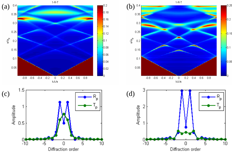
Rysunek 6.4. (a) i (b) Relacje dyspersji asymetrycznej dwuwarstwowej struktury o parametrach: d_1 = d_2 = 60nm , f_1 = f_2 = 0.4\Lambda , n_4 = 1 , n_5 = 1.5 oraz (c) i (d) unormowane amplitudy kolejnych rzędów ugięcia pola H_y dla d_x = 0\Lambda (lewa kolumna) i d_x = 0.5\Lambda (prawa kolumna).
