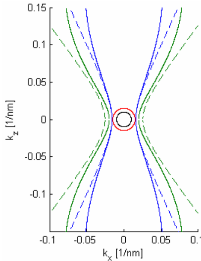
Rysunek 8.1. Analizytna zależność pomiędzy k_x i k_z dla częstotliwości \omega = 0.2157\omega_p w przypadku jednorodnego anizotropowego ośrodka o nieskończonej grubości charakteryzowanego przenikalnościami \epsilon_x i \epsilon_z obliczonymi dla parametrów: \epsilon_1 = 1 i \epsilon_2 = 1 - \omega_p^2/\omega^2 (niebieska przerywana linia) oraz \epsilon_1 = 2.25 i \epsilon_2 = 1 - \omega_p^2/\omega^2 (zielona przerywana linia), a także zależność dla powietrza \epsilon = 1 (czarna linia) i dielektryka \epsilon = 2.25 (czerwona linia). Ciągłe krzywe: zależność dla analogicznych struktur periodycznych o skończonych grubościach warstw ( d_1 \approx 7\text{nm} , d_2 \approx 11\text{nm} ).
