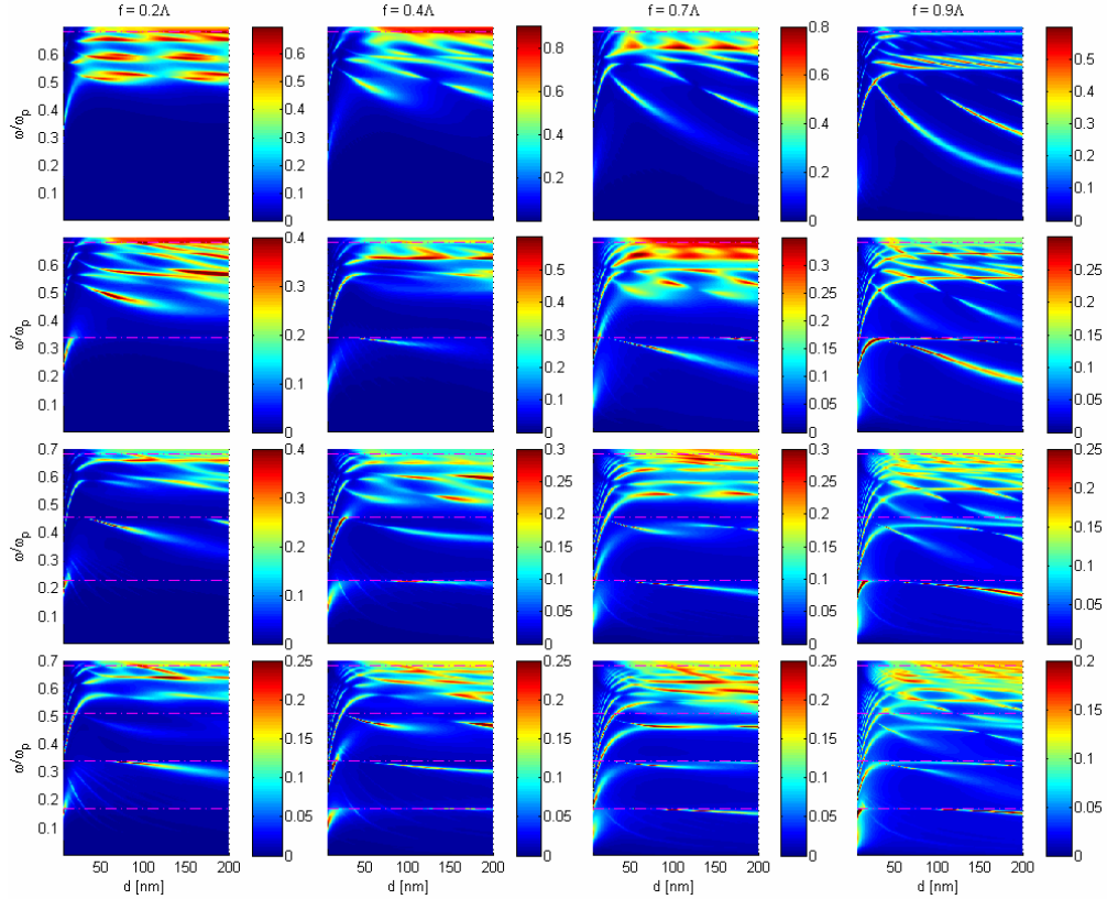
Rysunek 7.7. Zależność absorpcji ( A=1-R-T ) od częstotliwości fali padającej normalnie i grubości siatki w jednorodnym, symetrycznym otoczeniu dielektrycznym ( n_1 = n_4 = n_3 = 1 ) dla zmiennych okresów (w rzędach z góry na dół: \Lambda = 200nm , 400nm , 600nm , 800nm ) oraz wypełnienia (w kolumnach od lewej do prawej: f = 0.2\Lambda , 0.4\Lambda , 0.7\Lambda , 0.9\Lambda ).
