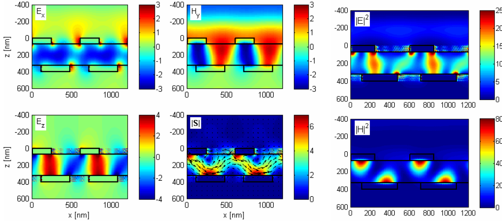
Rysunek 7.30. Rozkład unormowanych niezerowych składowych pola EM oraz natężeń pola elektrycznego i magnetycznego w otoczeniu siatki o okresie \Lambda = 600\text{nm} , wypełnieniu f_1 = 0.4\Lambda i f_2 = 0.6\Lambda oraz przesunięciu d_x = 0.283\Lambda , grubość dielektryka: d_{\text{diel}} = 250\text{nm} , \omega = 0.156\omega_p , współczynniki załamania dielektryków: n_1 = n_3 = n_4 = n_5 = 1 , n_{\text{diel}} = 1.5 .
