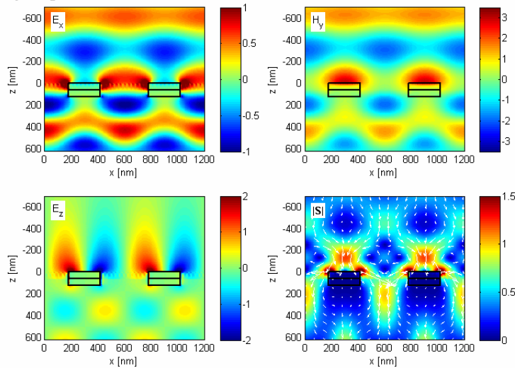
Rysunek 6.2. Unormowane amplitudy niezerowych składowych pola elektromagnetycznego: E_x , H_y , E_z oraz wartość i kierunek wypadkowego wektora Poyntinga |S| w pobliżu symetrycznej dwuwarstwowej struktury o parametrach: d_x = 0 , d_1 = d_2 = 60\text{nm} , f_1 = f_2 = 0.4\Lambda , n_4 = 1 , n_5 = 1.5 .
