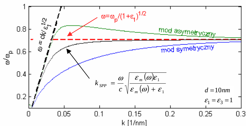
Rysunek 7.2. Dyspersja dla plazmonów powierzchniowych na warstwie metalu w symetrycznym otoczeniu. Czerwona przerywana prosta oznacza częstotliwość graniczną plazmonu na pojedynczej granicy. Czarna przerywana prosta jest linią dyspersji światła w powietrzu. Czarna krzywa – relacja dyspersji dla pojedynczej granicy (bądź bardzo grubej warstwy metalu), niebieska linia – mod symetryczny o niższej częstotliwości, zielona linia – mod asymetryczny o wyższej częstotliwości.
