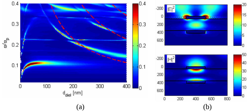
Rysunek 7.29. (a) Zależność częstości od grubości warstwy separującej dla układu dwóch siatek o okresie \Lambda = 800\text{nm} , wypełnieniu f_1 = f_2 = 0.3\Lambda i przesunięciu d_x = 0 . Przerywane krzywe wyznaczają analityczną zależność \omega(d_{\text{diel}}) dla kolejnych rezonansów we wnęce o skończonej długości. (b) Rozkłady natężenia pola elektrycznego i magnetycznego dla pierwszego modu wnękowego w strukturze ( d_{\text{diel}} = 300\text{nm} , \omega = 0.17\omega_p ).
