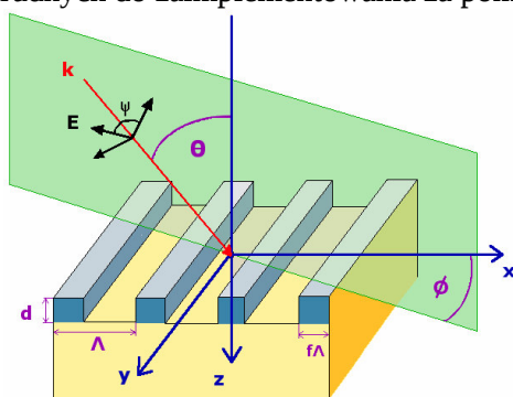
Rysunek 5.1. Schemat padania stożkowego (konikalnego) fali płaskiej o dowolnej polaryzacji liniowej na jednowarstwową strukturę periodyczną.
