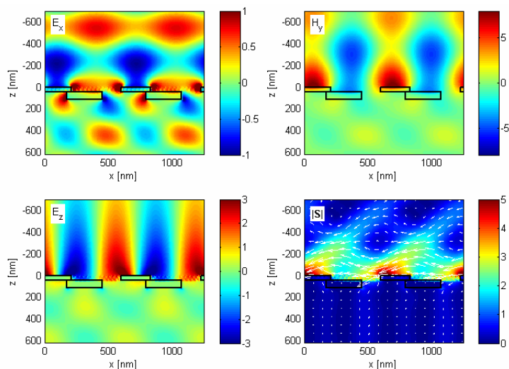
Rysunek 6.10. Unormowane amplitudy niezerowych składowych pola elektromagnetycznego: E_x , H_y , E_z oraz wartość i kierunek wypadkowego wektora Poyntinga |\underline{S}| w pobliżu asymetrycznej dwuwarstwowej struktury o parametrach: d_x = 0.35\Lambda , \Lambda = 624\text{nm} , d_1 = 46\text{nm} , d_2 = 70\text{nm} , f_1 = 0.372\Lambda , f_2 = 0.443\Lambda , n_4 = 1 , n_5 = 1.5 .
