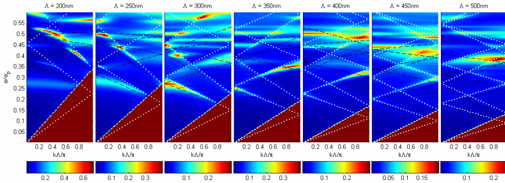
Rysunek 7.22. Zależność absorpcji od częstotliwości fali i wektora falowego dla struktur o okresach od \Lambda = 200\text{nm} do \Lambda = 500\text{nm} . Szerokość paska metalu w każdym z przypadków jest stała i równa 150\text{nm} , wysokość siatki: d = 120\text{nm} , współczynniki załamania: n_1 = n_4 = 1 , n_3 = 1.5 .
