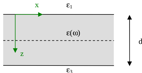
Rysunek 7.1. Schemat metalowej warstwy o grubości d i funkcji dielektrycznej \varepsilon(\omega) , otoczonej ośrodkami dielektrycznymi o różnych w ogólności współczynnikach załamania \varepsilon_1 i \varepsilon_3 .
