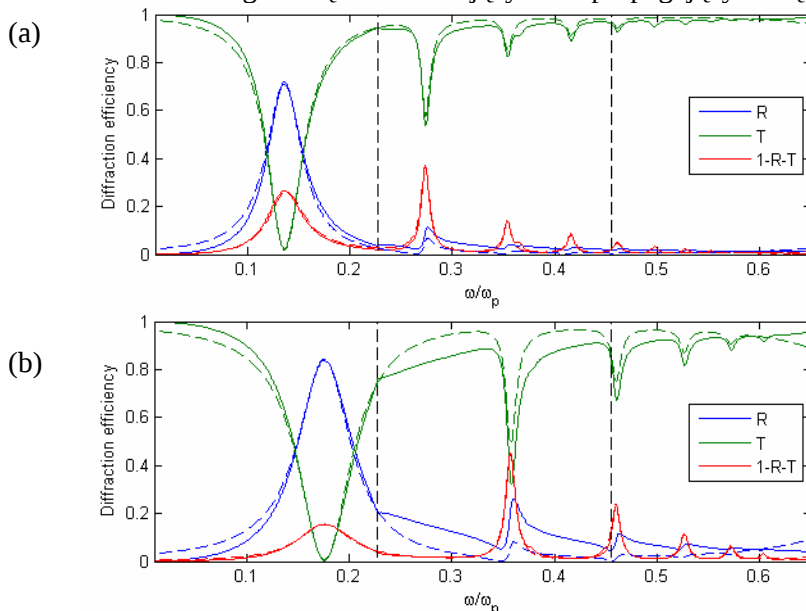
Rysunek 7.8. Ewolucja symetrycznych modów rezonansowych na paskach metalu o szerokości 240\text{nm} i ustawionych periodycznie, o okresie \Lambda = 600\text{nm} w jednorodnym otoczeniu dielektrycznym ( n_1 = n_4 = n_3 = 1 ), o różnych grubościach siatki: (a) d = 5\text{nm} , (b) d = 10\text{nm} . Linie ciągłe przedstawiają reflektancję, transmitancję i absorpcję obliczone za pomocą metody RCWA, natomiast linie przerywane zostały dopasowane za pomocą modelu fenomenologicznego. Pionowe linie wyznaczają częstotliwości anomalii Rayleigha.
