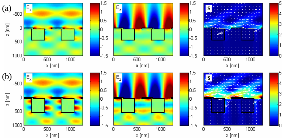
Rysunek 6.15. Unormowane amplitudy niezerowych składowych pola elektrycznego: E_x , E_z oraz wartość i kierunek wypadkowego wektora Poyntinga |\underline{S}| w pobliżu asymetrycznej dwuwarstwowej struktury o parametrach: d_x = 0.35\Lambda , \Lambda = 624\text{nm} , d_1 = 46\text{nm} , f_1 = 0.372\Lambda , f_2 = 0.443\Lambda , n_4 = n_5 = 1.5 oraz (a) d_2 = 400\text{nm} , (b) d_2 = 501\text{nm} . Skale kolorów na odpowiadających sobie wykresach w obu przypadkach są takie same.
