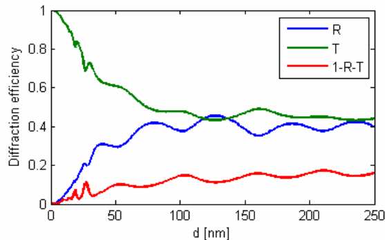
Rysunek 7.15. Zależność absorpcji od grubości siatki dla częstości fali padającej \omega = 0.652\omega_p w jednorodnym, symetrycznym otoczeniu dielektrycznym ( n_1 = n_4 = n_3 = 1 ). Okres \Lambda = 600\text{nm} , wypełnienie struktury f = 0.4\Lambda .
