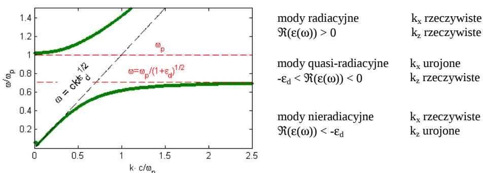
Rysunek 4.3. Relacja dyspersji dla granicy między metalem a dielektrykiem dla \epsilon_d = 1 .
