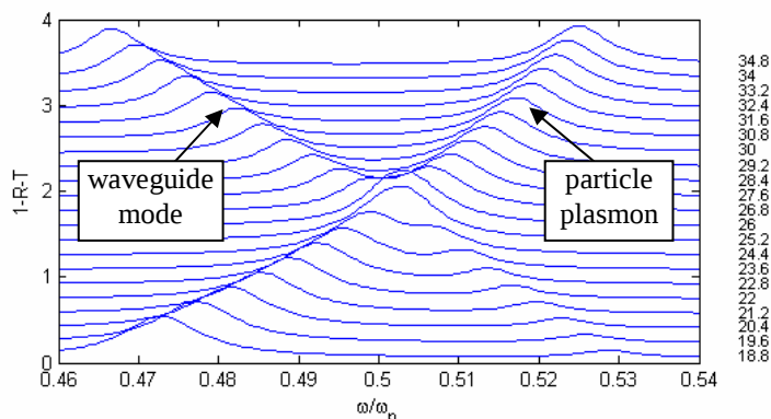
Rysunek 7.17. Zależność częstotliwości od grubości siatki w jednorodnym, symetrycznym otoczeniu dielektrycznym ( n_1 = n_4 = n_3 = 1 ). Okres \Lambda = 200\text{nm} , wypełnienie struktury f = 0.9\Lambda .
