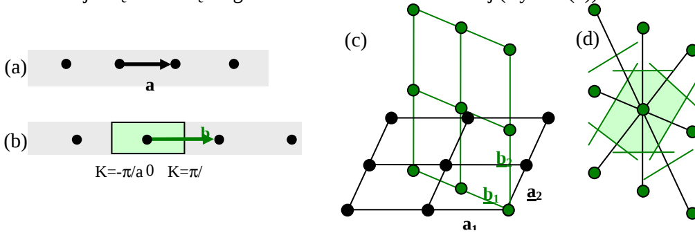
Rysunek 4.1. (a) Jednowymiarowa sieć prosta oraz (b) jej sieć odwrotna. Granice pierwszej strefy Brillouina jednowymiarowej sieci odwrotnej określone są przez wartości wektorów \underline{K} = \pm\pi/\underline{a} , gdzie \underline{a} jest stałą sieci prostej kryształu. (c) Sieć prosta ( \underline{a}_1 , \underline{a}_2 ) i odwrotna ( \underline{b}_1 , \underline{b}_2 ) dwuwymiarowej sieci ukośnej. (d) Komórka elementarna Wignera-Seitza dwuwymiarowej ukośnej sieci odwrotnej.
