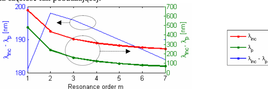
Rysunek 7.14. Długości fali wzbudzającej, długości fali plazmonów oraz ich różnica w przypadku kolejnych rezonansów modu symetrycznego w falowodzie IMI o grubości d = 10\text{nm} .
