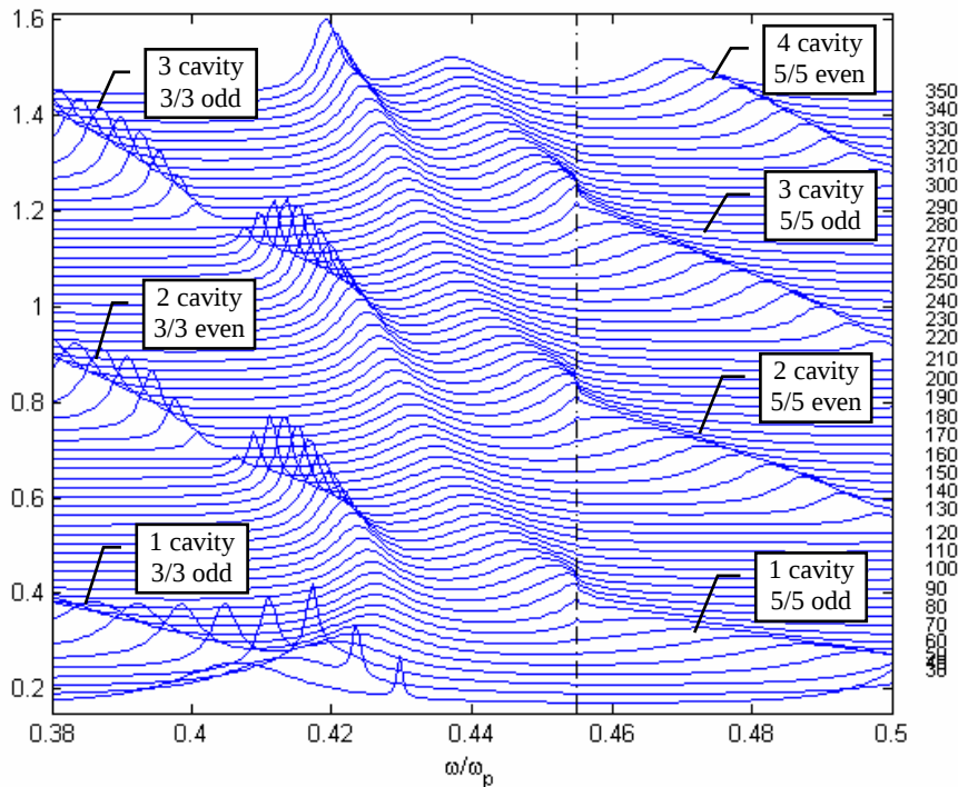
Rysunek 7.20. Zależność częstości fali padającej \omega od grubości siatki w jednorodnym, symetrycznym otoczeniu dielektrycznym ( n_1 = n_4 = n_3 = 1 ). Okres \Lambda = 600\text{nm} , wypełnienie struktury f = 0.9\Lambda . Po prawej stronie oznaczono co drugą wartość grubości siatki d [nm].
