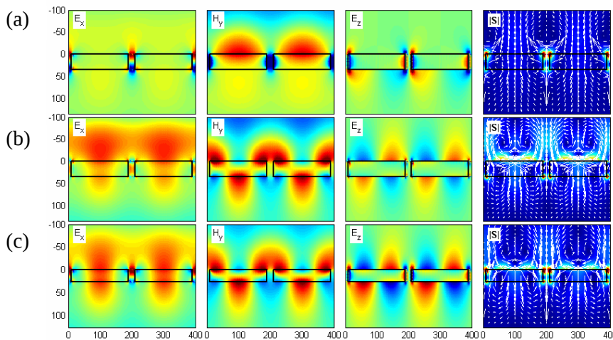
Rysunek 7.18. Rozkłady unormowanych amplitud składowych pól E_x , H_y i E_z oraz wartość i kierunek wektora Poyntinga dla (a) rezonansu cząsteczkowego i (b) modu wnątkowego przy stałej grubości siatki d = 34.8 \text{ nm} oraz (c) złożenie obu rezonansów dla d = 25.2 \text{ nm} . Okres siatki \Lambda = 200 \text{ nm} , wypełnienie struktury f = 0.9\Lambda , jednorodne, symetryczne otoczenie dielektryczne ( n_1 = n_4 = n_3 = 1 ).
