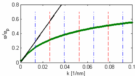
Rysunek 7.13. Analityczna relacja dyspersji modu symetrycznego w falowodzie IMI o grubości d = 10\text{nm} . Czarna prosta – linia dyspersji dla światła. Pionowe przerywane linie oznaczają wartości wektora k dla kolejnych nieparzystych (niebieskie) i parzystych (czerwone) rezonansów.
