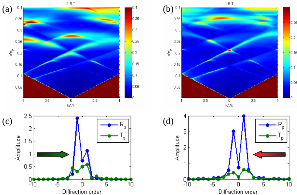
Rysunek 6.11. (a) i (b) Relacje dyspersji asymetrycznej dwuwarstwowej struktury o przesunięciu d_x = 0.35\Lambda i parametrach: \Lambda = 624nm , d_1 = 46nm , d_2 = 70nm , f_1 = 0.372\Lambda , f_2 = 0.443\Lambda , oraz (c) i (d) unormowane amplitudy kolejnych rzędów ugięcia pola H_y dla n_4 = n_5 = 1.5 (lewa kolumna) i n_4 = 1 , n_5 = 1.5 (prawa kolumna).
