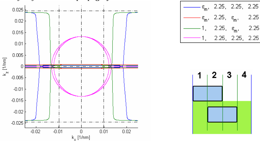
Rysunek 8.2. Zależność pomiędzy k_x i k_z dla częstotliwości \omega = 0.2157\omega_p dla czterech jednorodnych w kierunku x warstwowych struktur o układzie warstw odpowiadającym obszarom zaznaczonym na schemacie po prawej i o grubościach odpowiadających przypadkowi przesunięcia horyzontalnego. Grubość warstwy dielektryka pomiędzy siatkami wynosi d_{diel} = 2nm .
