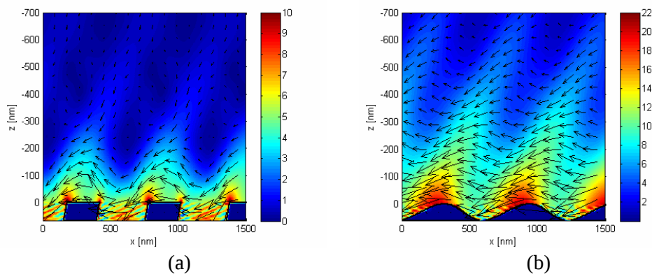
Rysunek 1.4. Wartość i kierunek uśrednionego w czasie wektora Poyntinga dla jednokierunkowej propagacji SPP wzdłuż nachylonych metalowych siatek dyfrakcyjnych o profilu (a) prostokątnym i (b) sinusoidalnym w reżimie padania normalnego (na podst. [57]).
