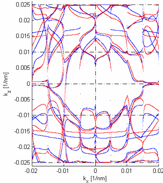
Rysunek 8.4. Zależność pomiędzy k_x i k_z dla częstości \omega = 0.2157\omega_p (niebieskie linie) oraz \omega = 0.22\omega_p (czerwone linie) w przypadku struktury odpowiadającej asymetrii horyzontalnej dla przesunięcia d_x = 0.35\lambda dla trzech rzędów ugięcia.
