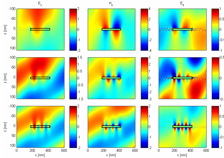
Rysunek 7.12. Unormowane amplitudy składowych E_x , H_y i E_z dla trzech pierwszych parzystych rezonansów dla grubości siatki d=10\text{nm} na granicy strefy Brillouina w jednorodnym, symetrycznym otoczeniu dielektrycznym ( n_1 = n_4 = n_3 = 1 ). Wypełnienie struktury f=0.4\Lambda .
