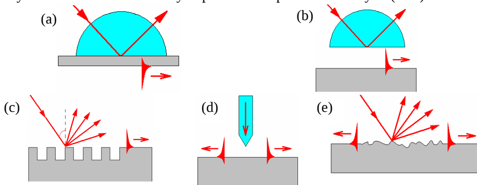
Rysunek 4.6. Różne metody wzbudzenia plazmonów polarytonów powierzchniowych: (a) konfiguracja Kretschmanna, (b) konfiguracja Otto, (c) wzbudzenie na siatce dyfrakcyjnej, (d) lokalne wzbudzenie za pomocą sondy SNOM, (e) nierezonansowe wzbudzenie na niejednorodnościach powierzchni.
