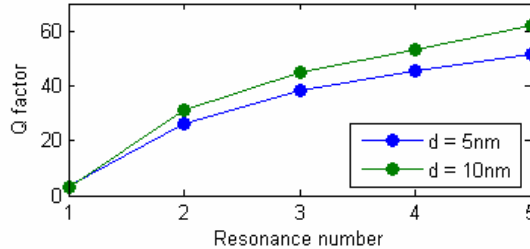
Rysunek 7.9. Dobroć Q pierwszych pięciu symetrycznych rezonansów na paskach metalu o szerokości 240\text{nm} , ustawionych periodycznie o okresie \Lambda = 600\text{nm} w jednorodnym otoczeniu dielektrycznym ( n_1 = n_4 = n_3 = 1 ), grubości siatek: d = 5\text{nm} i d = 10\text{nm} .
