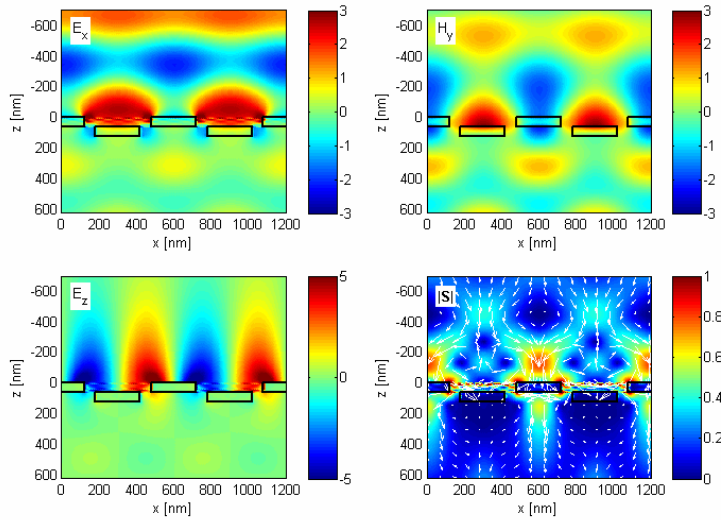
Rysunek 6.3. Unormowane amplitudy niezerowych składowych pola elektromagnetycznego: E_x , H_y , E_z oraz wartość i kierunek wypadkowego wektora Poyntinga |S| w pobliżu symetrycznej dwuwarstwowej struktury o parametrach: d_x = 0.5\Lambda , d_1 = d_2 = 60\text{nm} , f_1 = f_2 = 0.4\Lambda , n_4 = 1 , n_5 = 1.5 .
