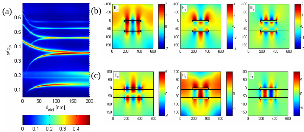
Rysunek 7.28. (a) Zależność częstości od grubości warstwy dielektryka dla d_1 = d_2 = 10\text{nm} , \Lambda = 600\text{nm} , f_1 = f_2 = 0.4\Lambda . (b) i (c) Unormowane amplitudy składowych E_x , H_y i E_z dla modu parzystego ( \omega = 0.384\omega_p ) i nieparzystego ( \omega = 0.326\omega_p ) dla d_{\text{diel}} = 50\text{nm} w jednorodnym, symetrycznym otoczeniu dielektrycznym ( n_1 = n_4 = n_3 = 1 ).
