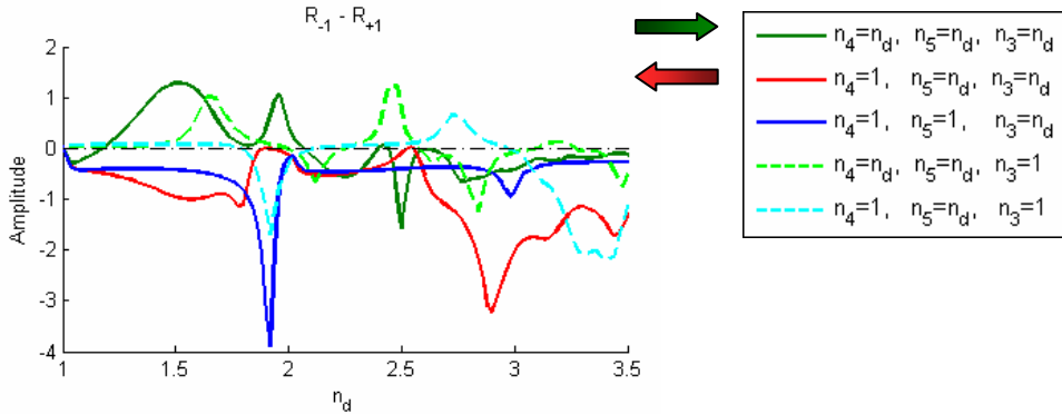
Rysunek 6.12. Różnica modułów amplitud -1 i +1 odbitego rzędu ugięcia \Delta w zależności od współczynnika załamania wypełniającego strukturę n_d . Ciągłe linie: struktury na podłożu n_3 > 1 , kreskowane linie: struktury na podłożu n_3 = 1 . Parametry siatki: \Lambda = 624\text{nm} , d_1 = 46\text{nm} , d_2 = 70\text{nm} , f_1 = 0.372\Lambda , f_2 = 0.443\Lambda .
